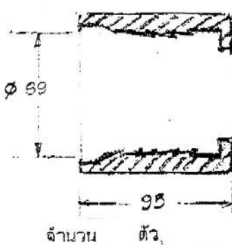
7) SLEEVE 3" (MS-48)
