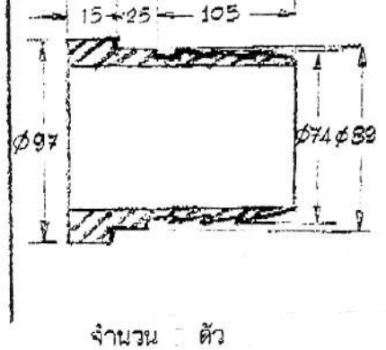
9) 3" INSERT
