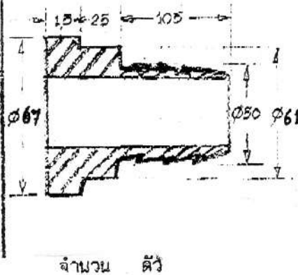
8) 2" INSERT
